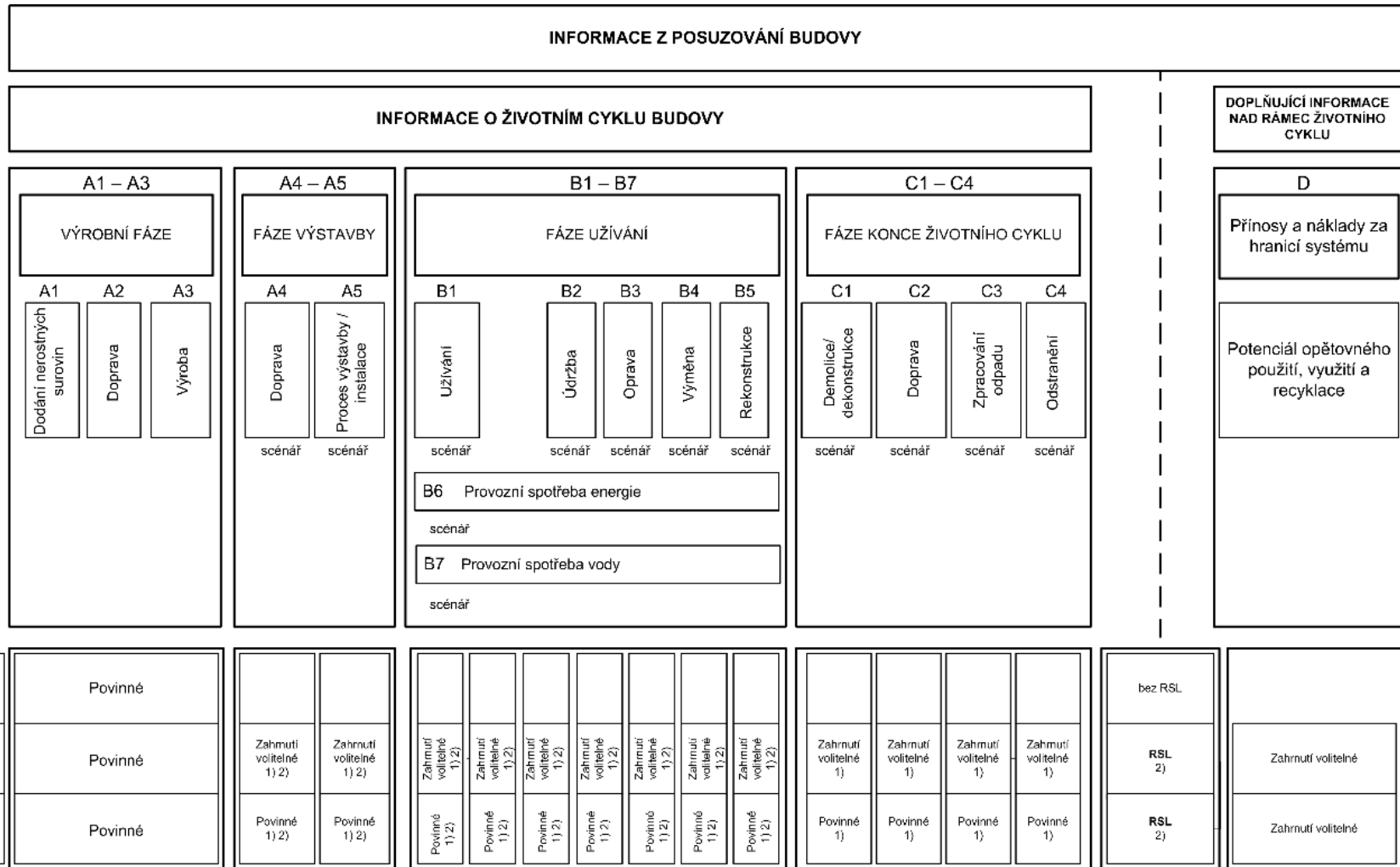
Obr. 14 Hranice systému dle ČSN EN 15804 [16]
